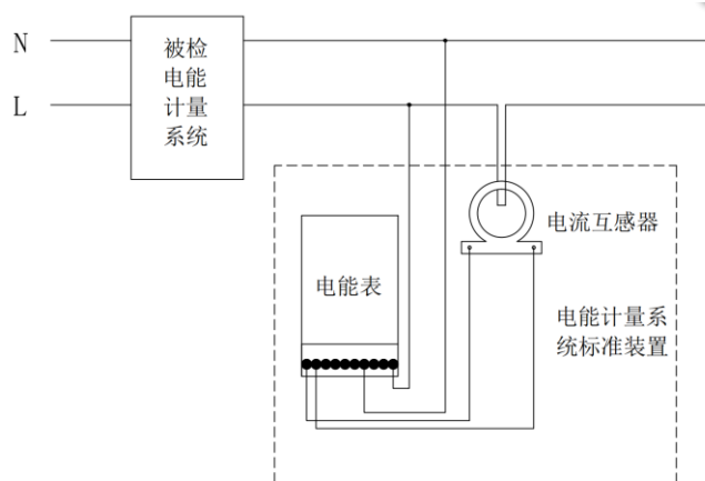
(b) 单相电能计量系统
