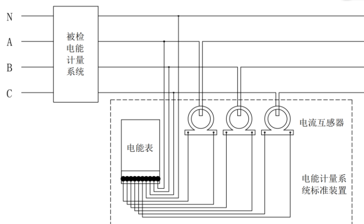
(a) 三相电能计量系统
